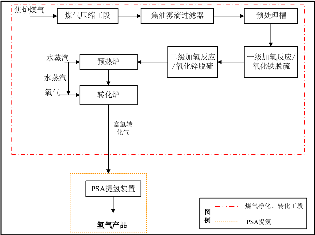
图 3-6 甲醇合成气 PSA 提氢项目
