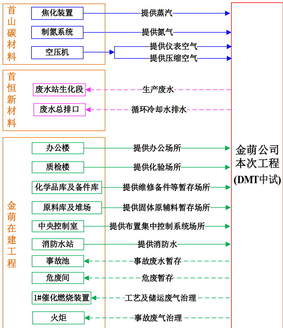
图 3-2 本项目与依托企业及依托工程关系图
