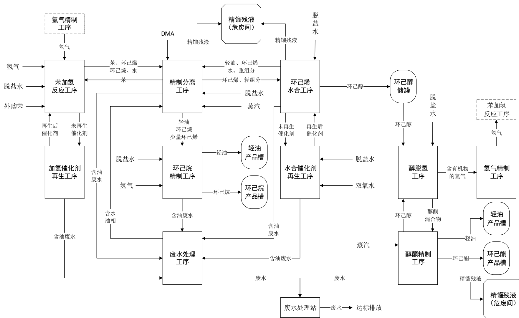
图 3-7 首恒新材料工艺流程图
