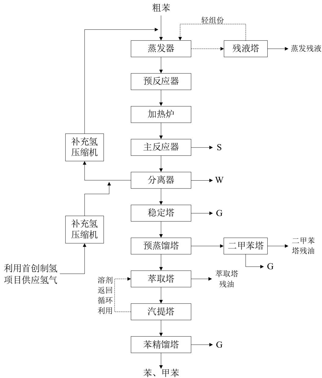
图 3-4 首创化工苯加氢项目生产工艺流程及产污环节
