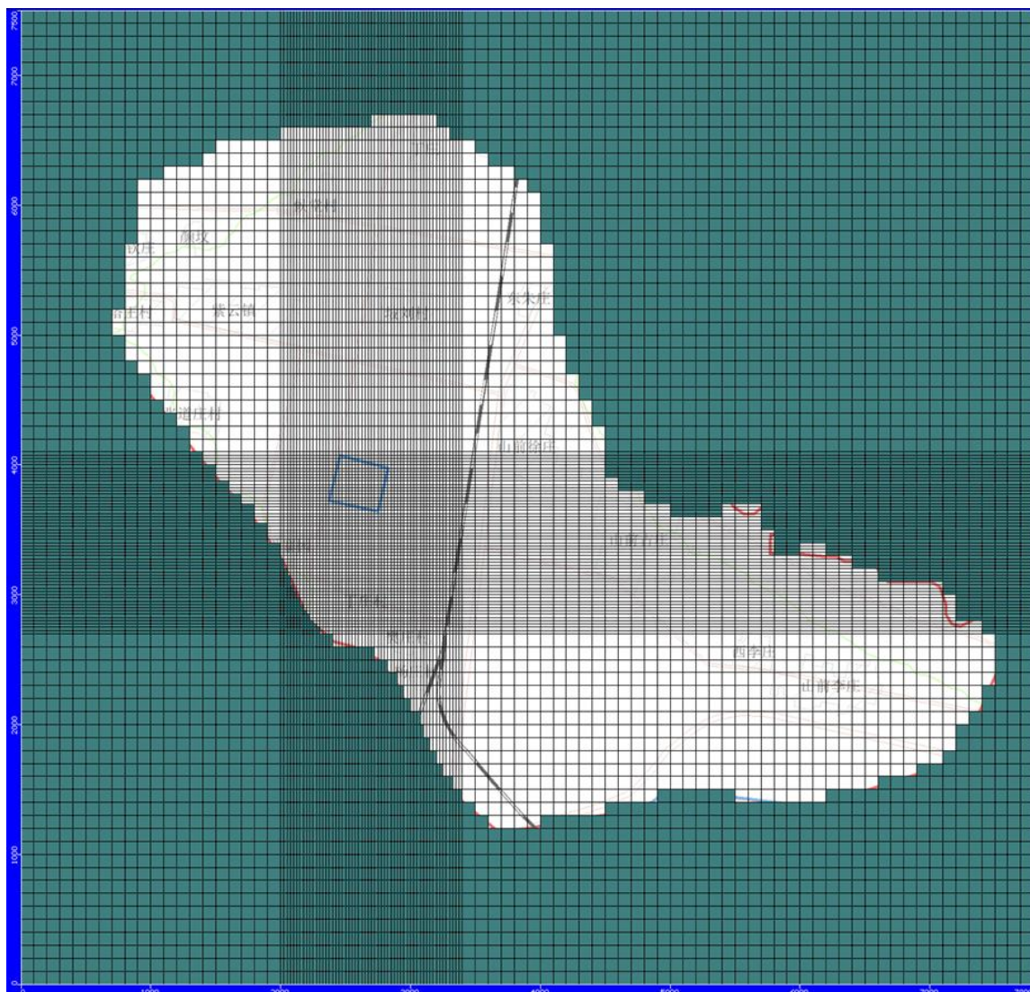
图 5-25 网格剖分
