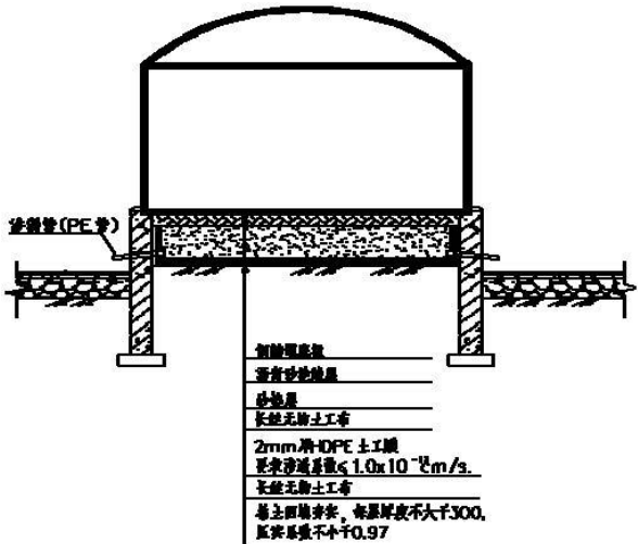
图 6-10 环墙式罐基础防渗
