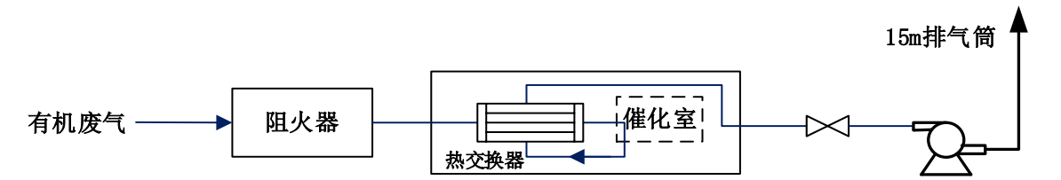
图 6-4 RCO 处理装置示意图
