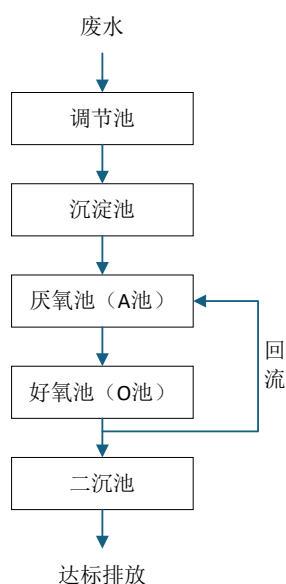
图 5-11 本项目废水处理站工艺流程图
