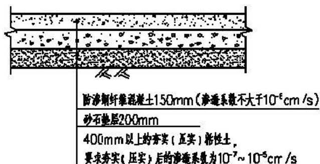
图 6-7 一般污染防治区地面防渗
