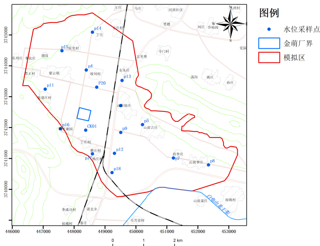
图 5-21 调查评价水位监测点示意图
