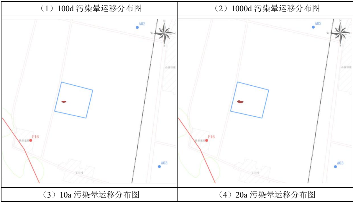
图 5-32 污染晕迁移分布图（石油类）
