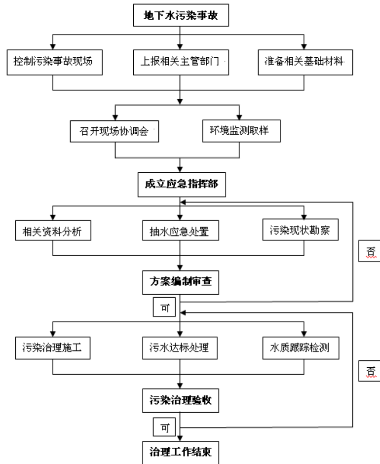
图 6-12 地下水污染应急治理程序框图
