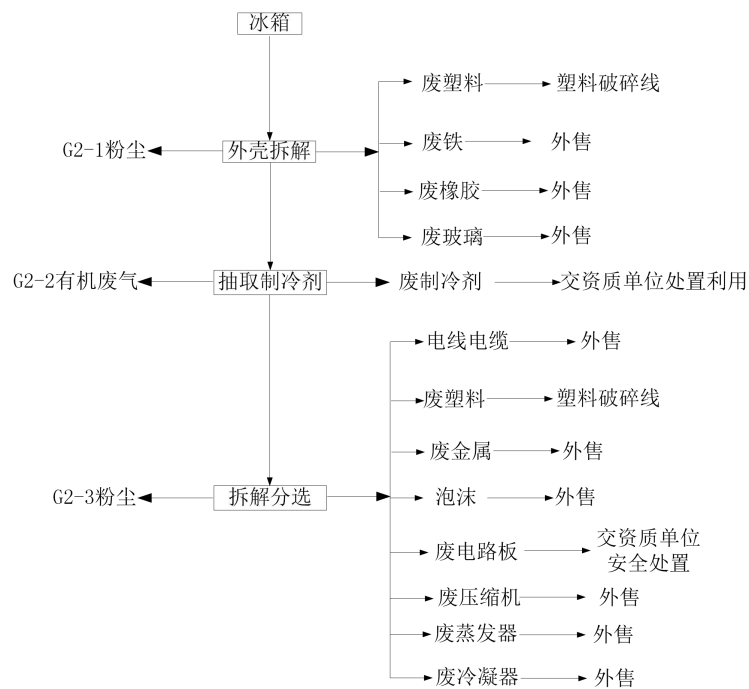
图 2-4 废冰箱拆解生产工艺流程及产污环节图
