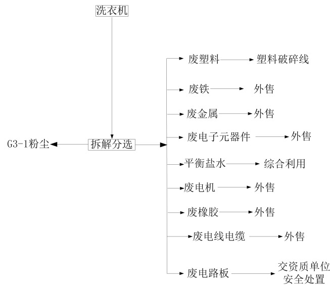
图 2-5 洗衣机拆解生产工艺流程及产污环节图
