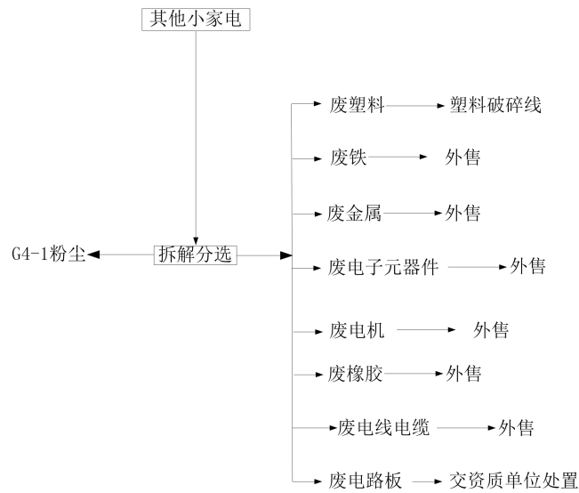
图 2-6 其他电器拆解生产工艺流程及产污环节图
