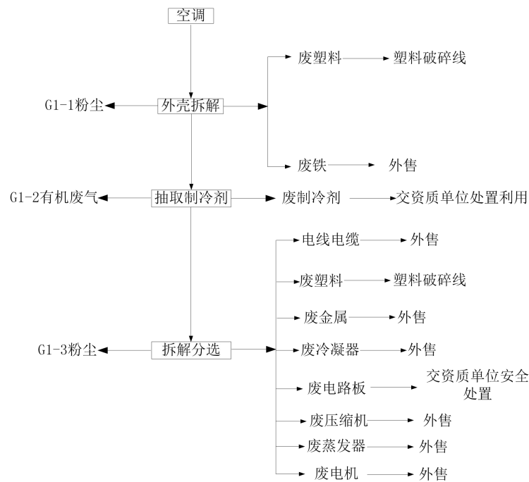
图 2-3 废空调拆解生产工艺流程及产污环节图
